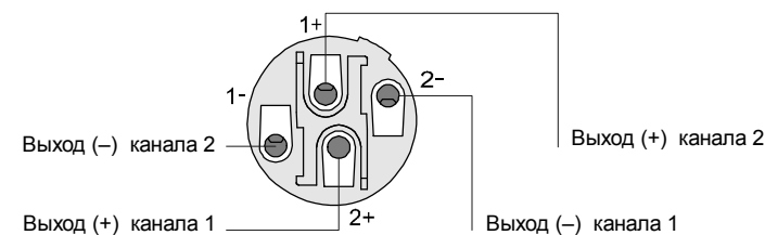
г) для подключения двух каналов одним соединителем (только соединитель канала 2)
