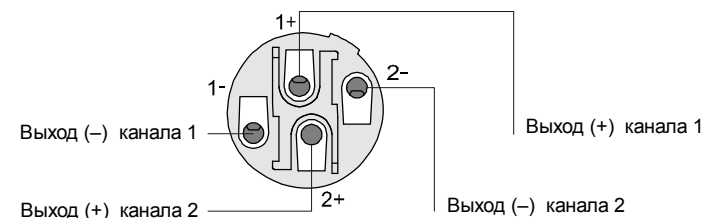
в) для подключения двух каналов одним соединителем (только соединитель канала 1)
